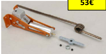
TREN PRINC.NEUMA.85° XPLANO. (VARILLAS) REF. 38123002
